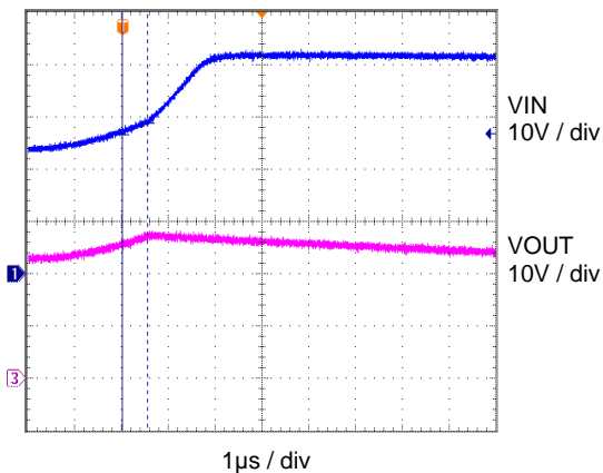
OVP Transient
