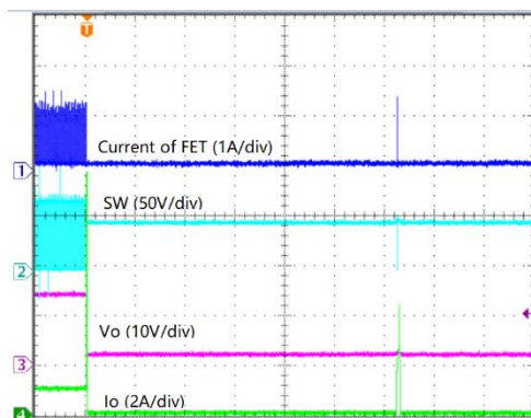
40ms / div
